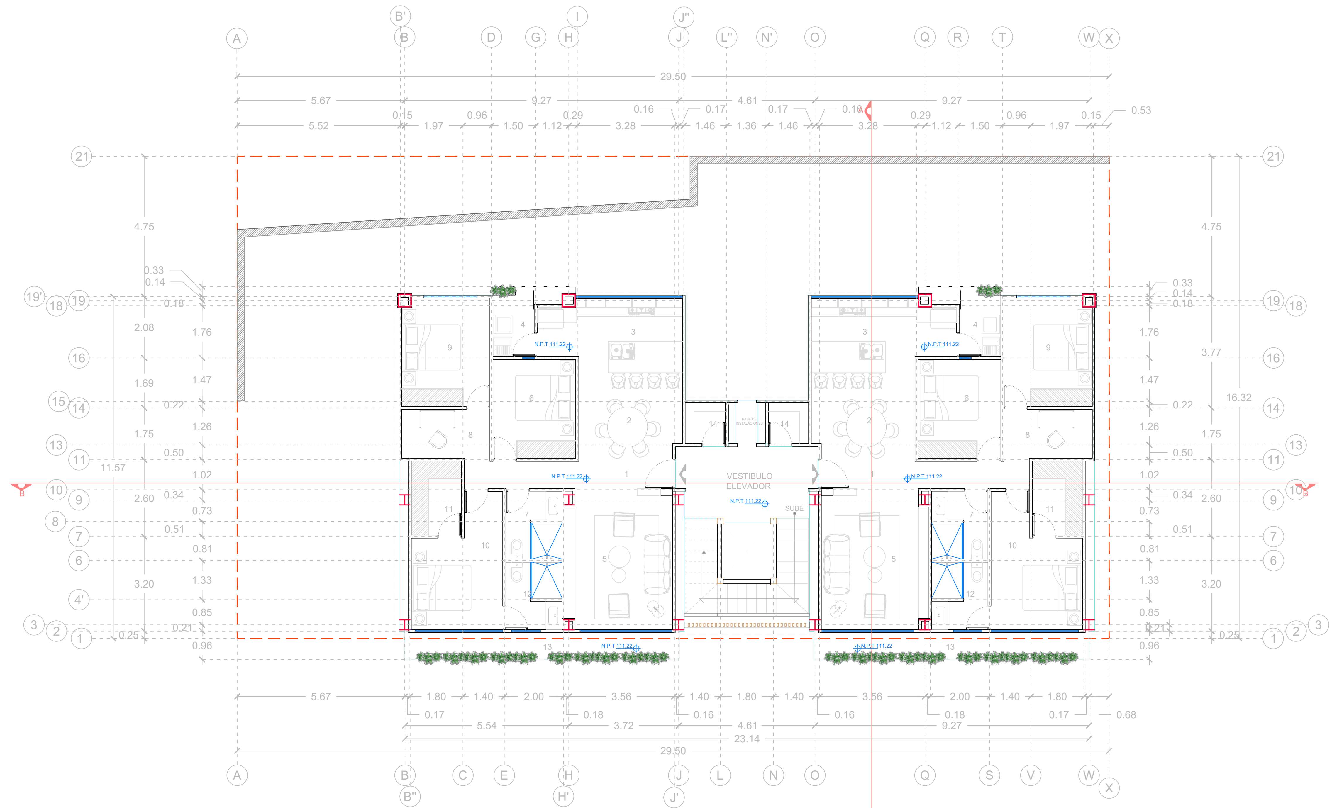
Planta Arquitectónica NIVEL 4
