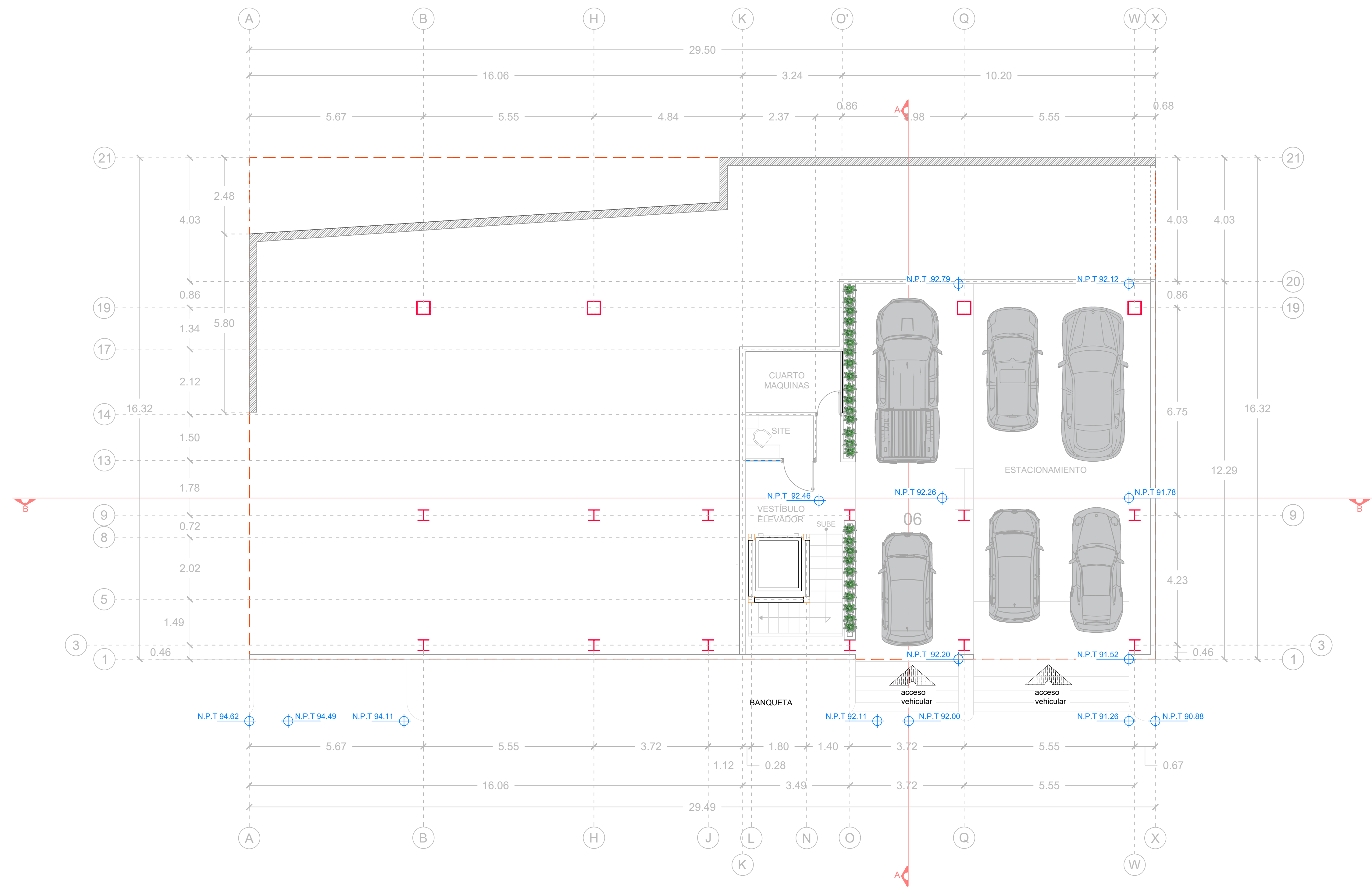
Planta Arquitectónica ESTACIONAMIENTO 1
