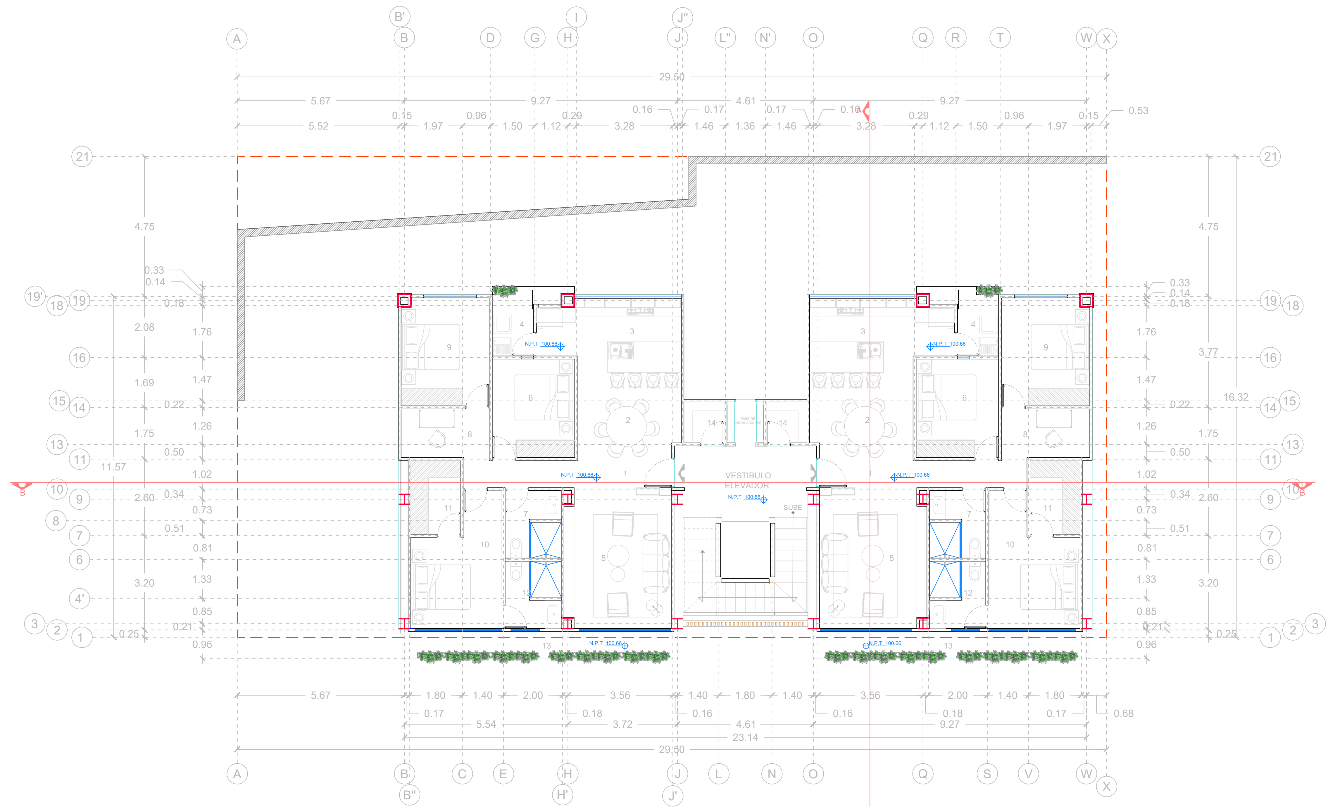
Planta Arquitectónica NIVEL 1
