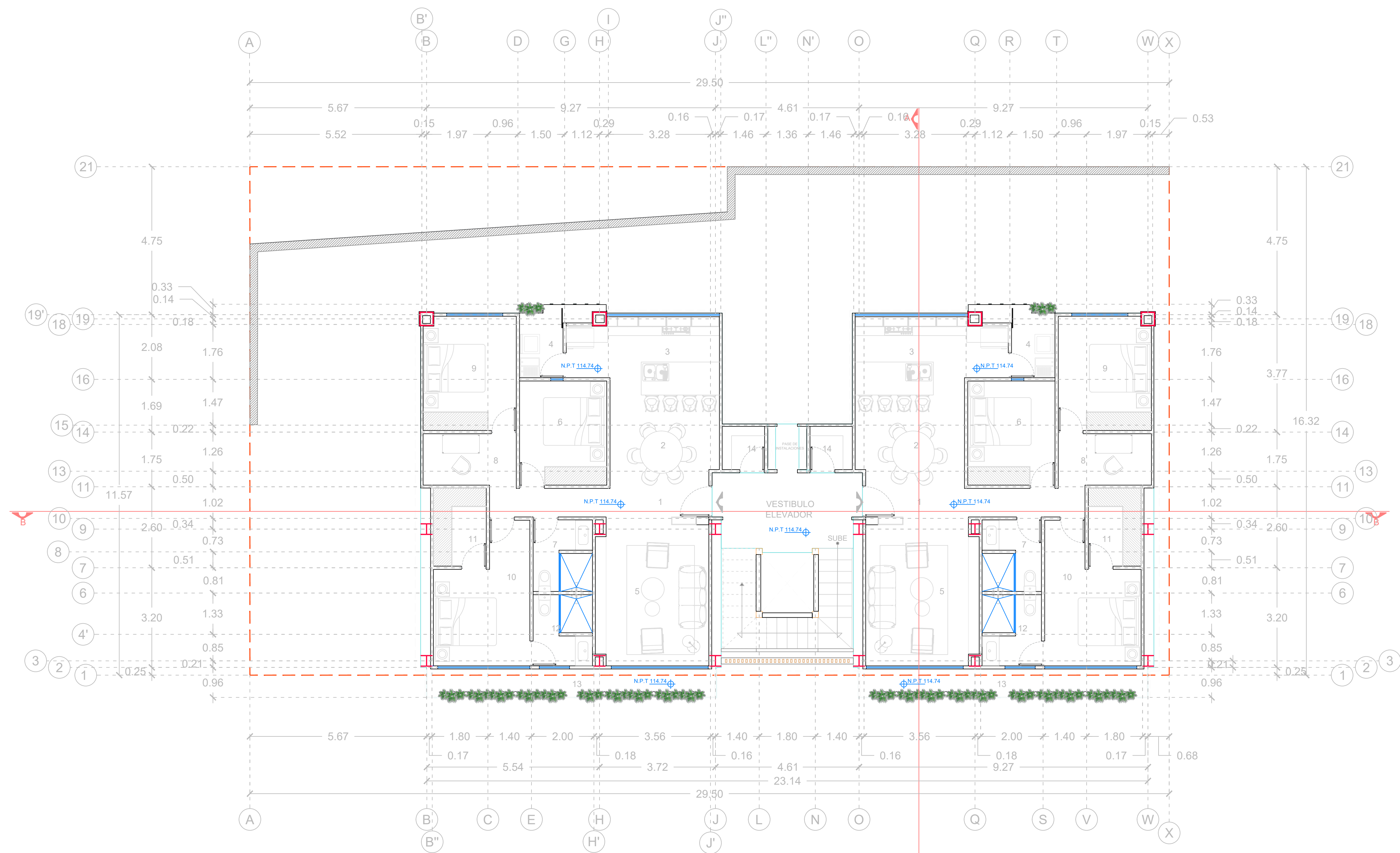
Planta Arquitectónica NIVEL 5
