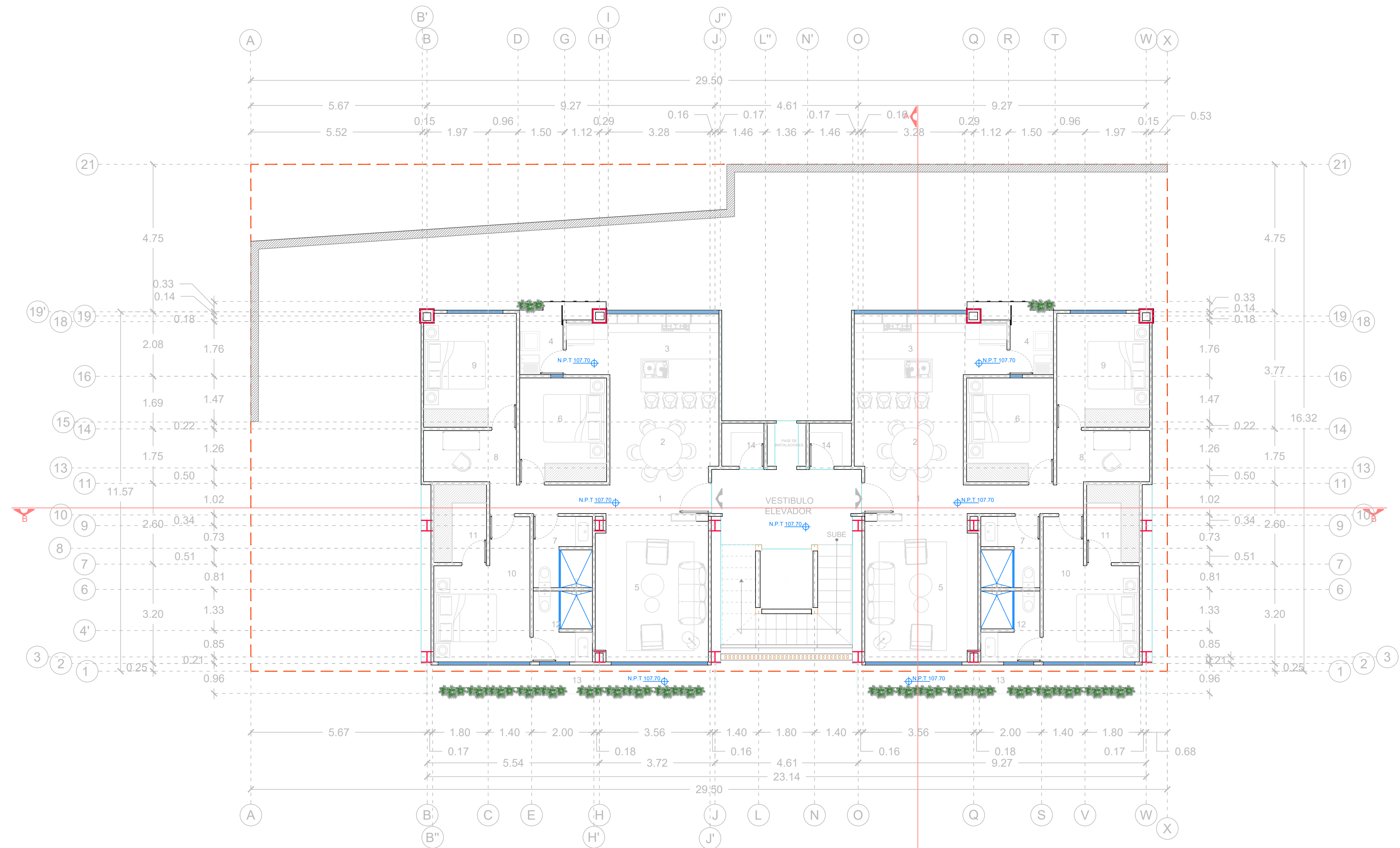
Planta Arquitectónica NIVEL 3
