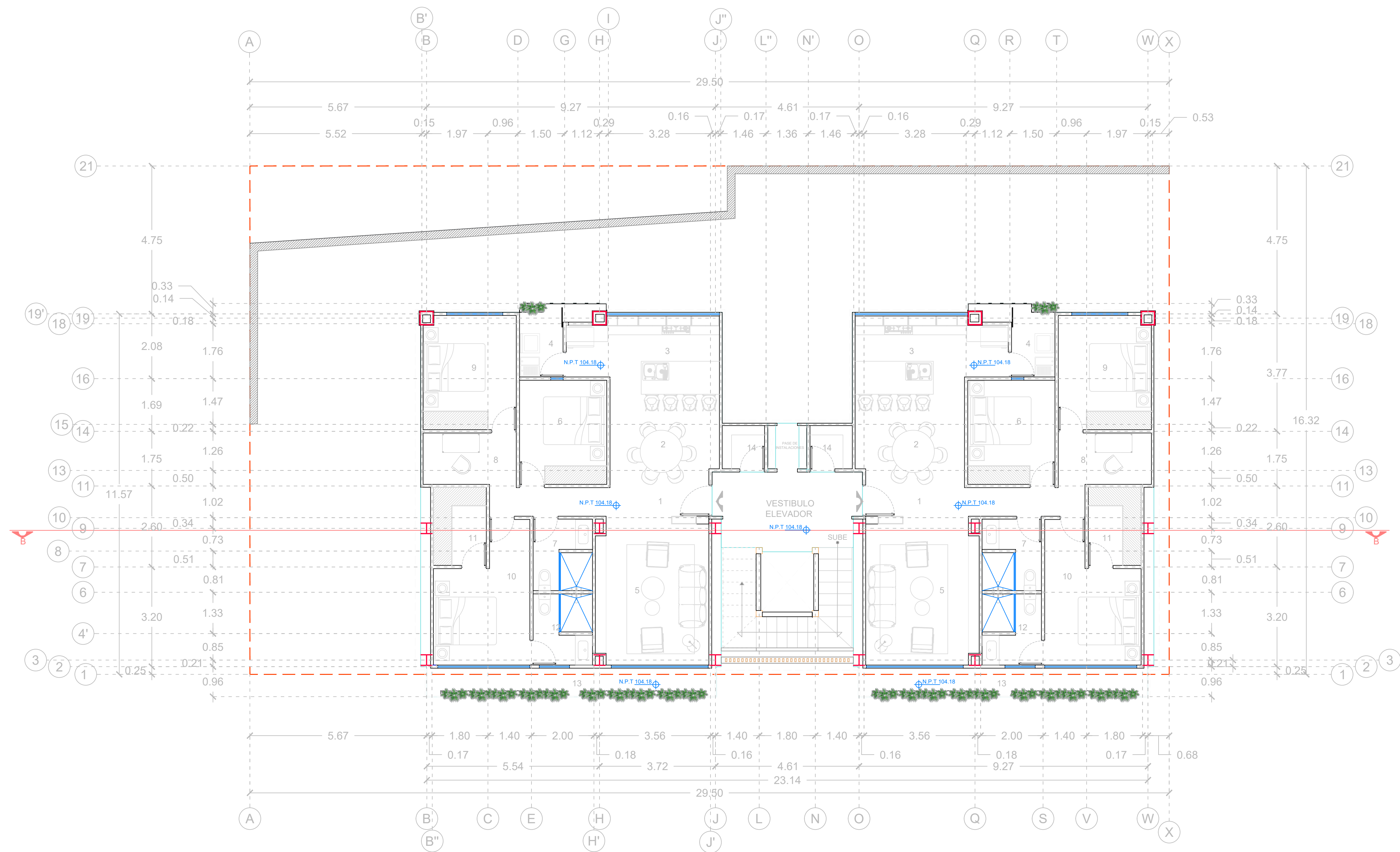
Planta Arquitectónica NIVEL 2
